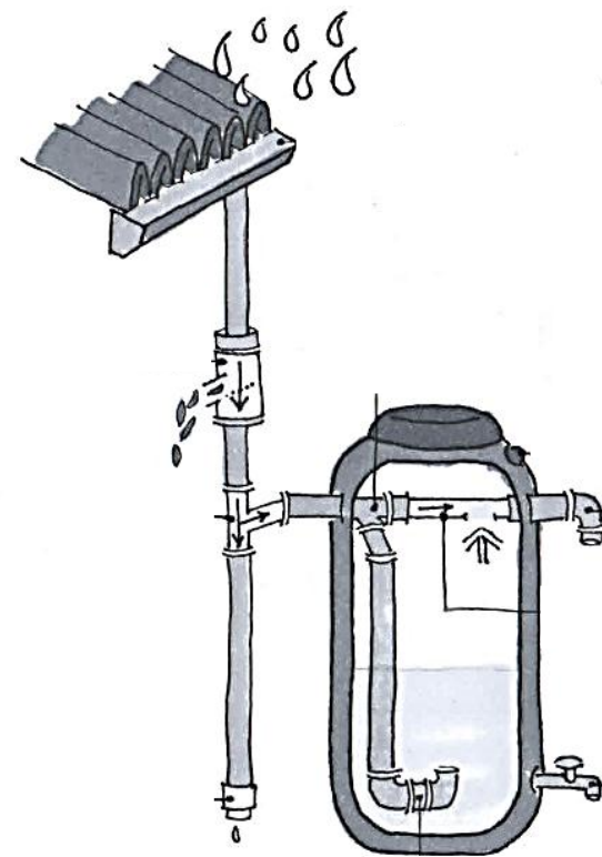
MINICISTERNA CASEIRA
