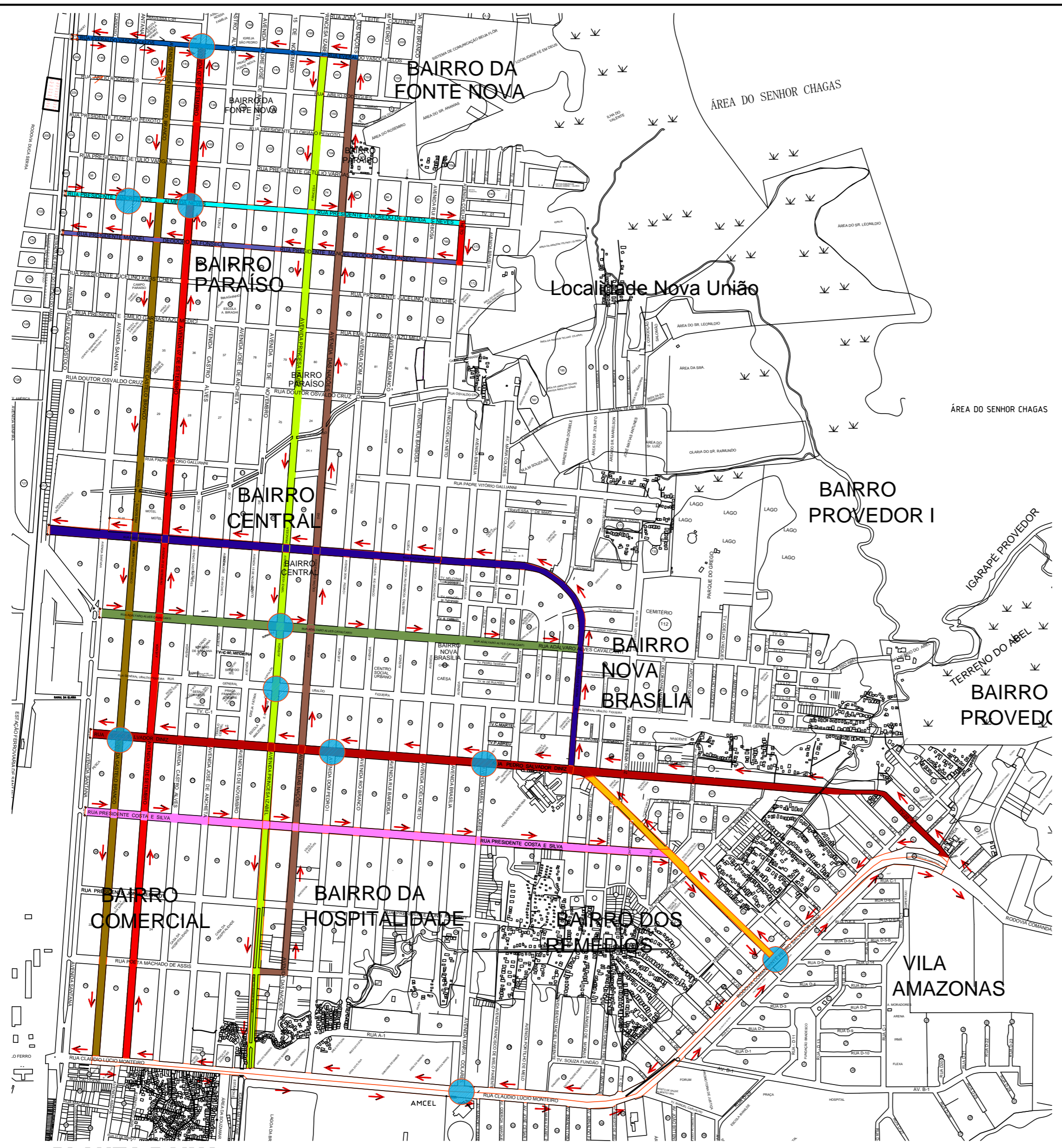
PLANTA BAIXA IMPLANTAÇÃO BINÁRIOS SEM ESC.
